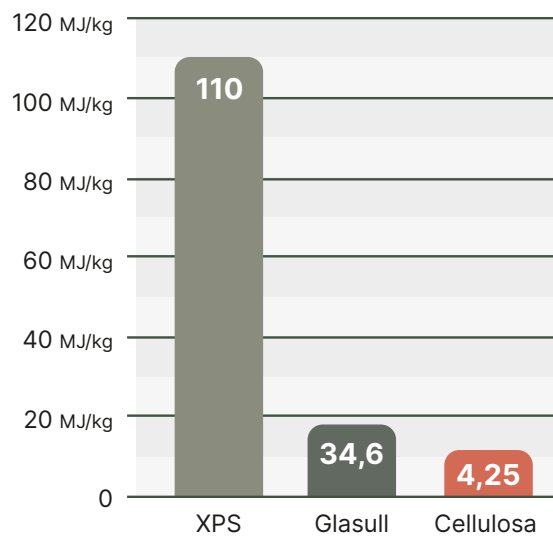
Jämförelse av premiärenergiuttag vid tillverkning av olika isoleringsmaterial:
